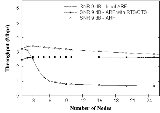
(b) SINR=9dB
